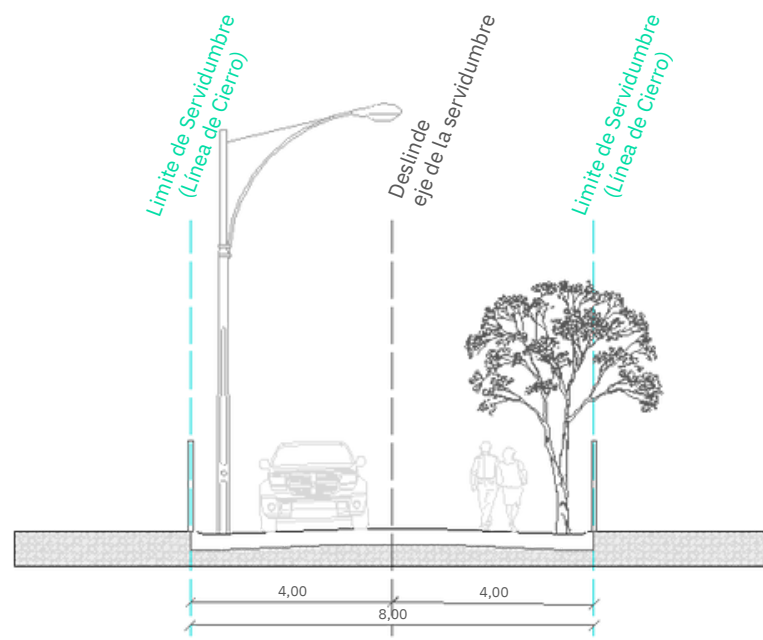
Perfil Servidumbre Esc. 1:150
